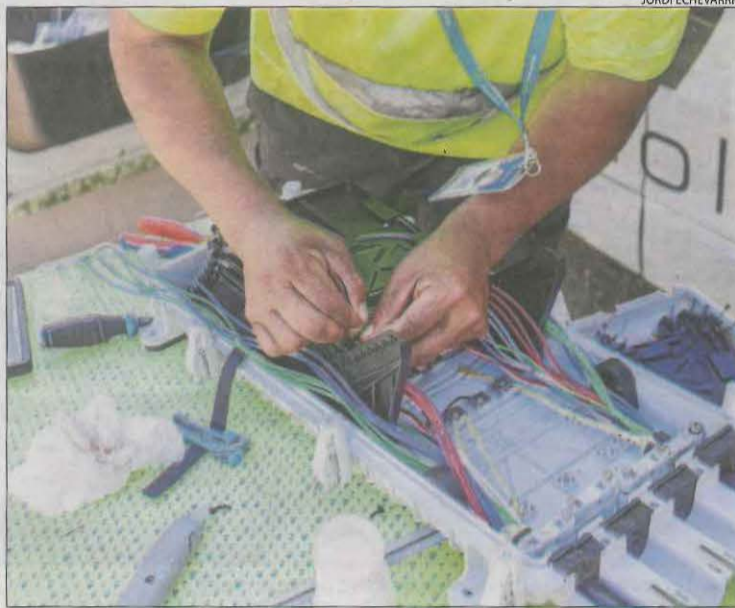
Els treballs per reparar els cables de fibra òptica danyats.
